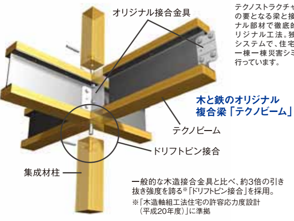
オリジナル接合金具 木と鉄のオリジナル 複合梁「テクノビーム」 テクノビーム ドリフトピン接合 集材材柱
